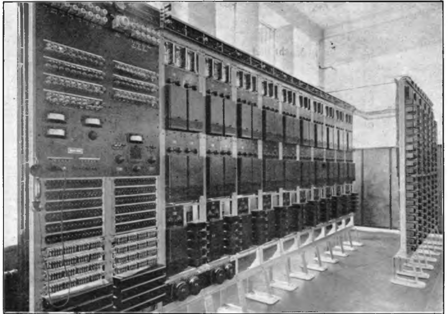
Paneelen met koordversterkers en controle-inrichting.
